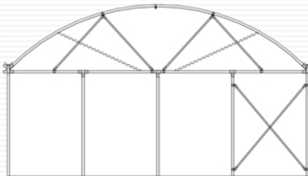
نمای قوس جلو و پشت Behind & Front Arcs Section
